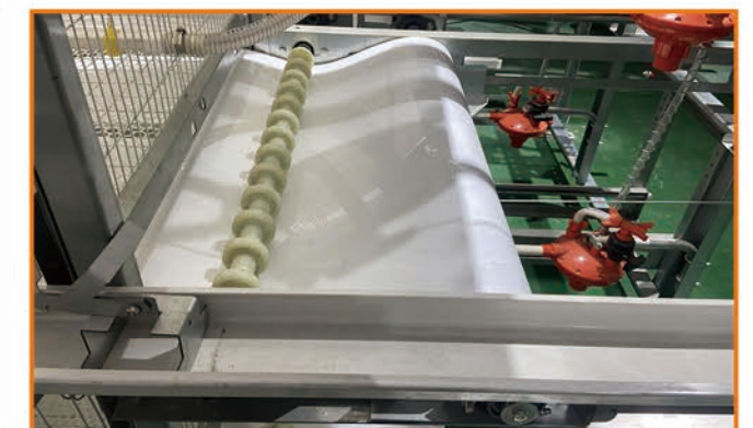
回料装置
