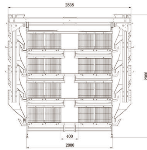
通风口尺寸400mm
