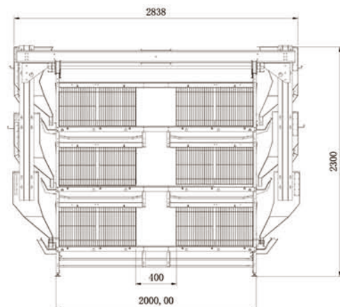
通风口尺寸400mm
