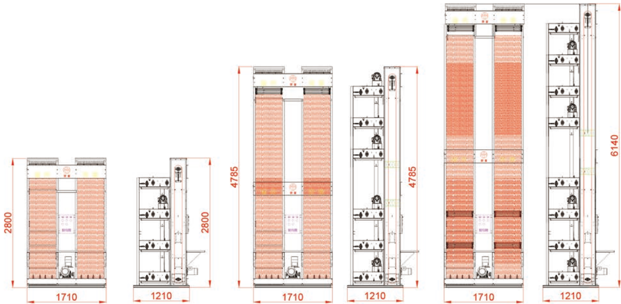
4层捡蛋机
